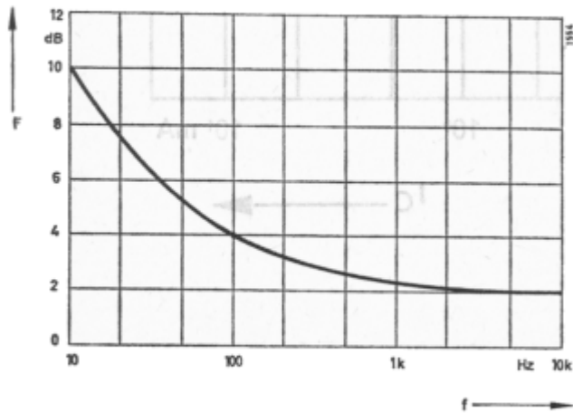
Rauschfaktor F = f(f) ; R_g = 10\text{ k}\Omega ; U_{CE} = 5\text{ V} ; I_C = 0,1\text{ mA} ; T_U = 25\text{ }^\circ\text{C} ; \Delta f = 1\text{ Hz}
