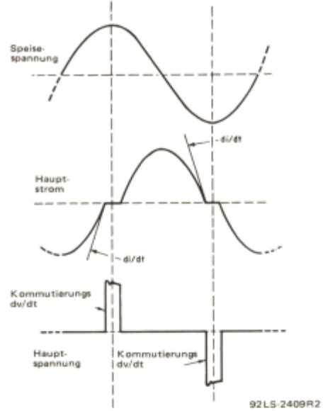
Bild 5 – Kommutierungs-Charakteristiken von Hauptstrom und -spannung
