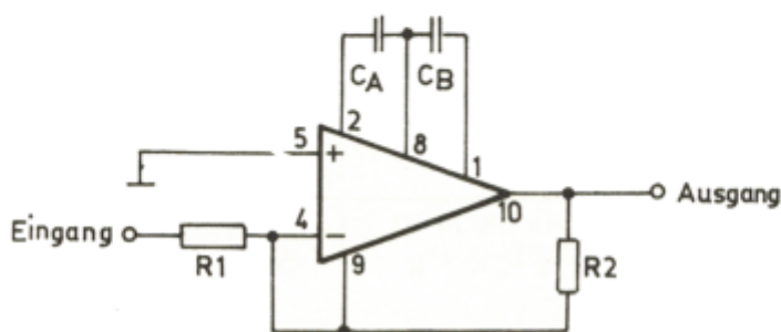
Applikationsschaltung: nichtinvertierender Verstärker
