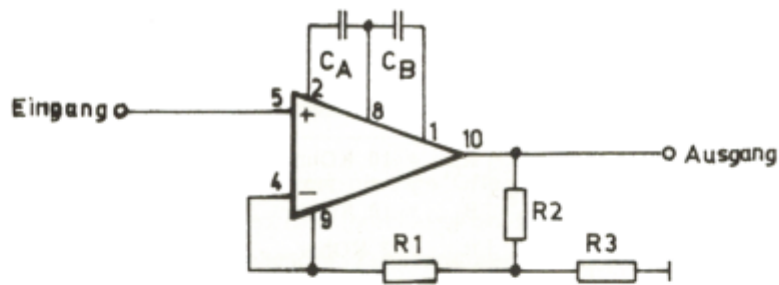
Applikationsschaltung: invertierender Verstärker
