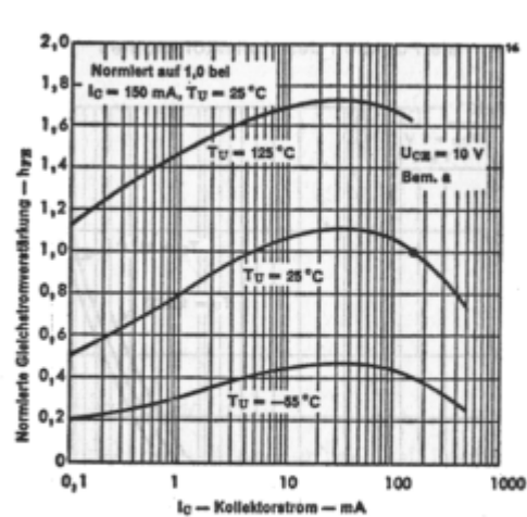
Normierte Gleichstromverstärkung als Funktion des Kollektorstromes
